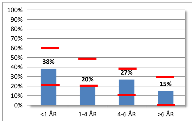
Räntebindning Kontokredit
