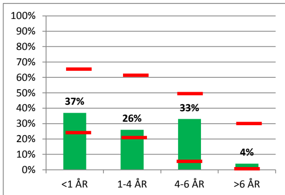
Kapitalbindning Kontokredit
